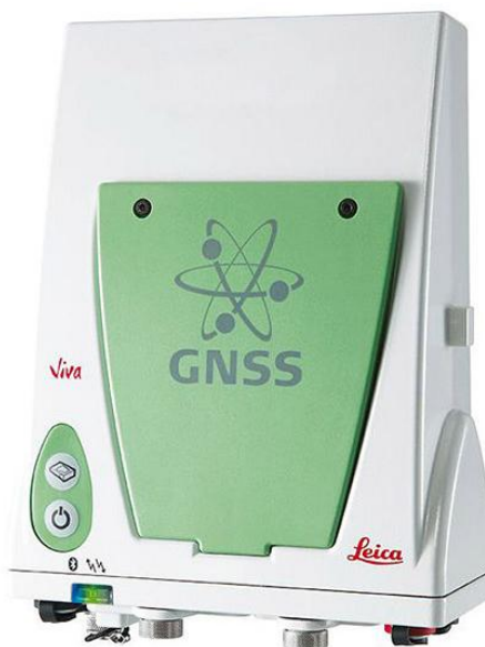
Рисунок 1 - Внешний вид аппаратуры геодезической спутниковой Leica GS10
